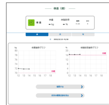
完了画面
