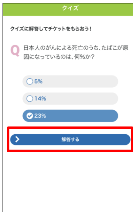
解答画面
