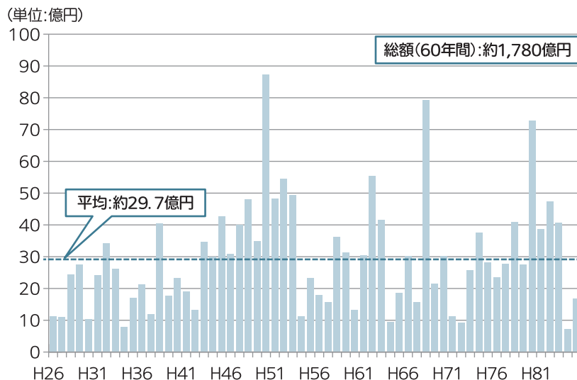
〔図③ 更新費用推計結果（60年間）〕
