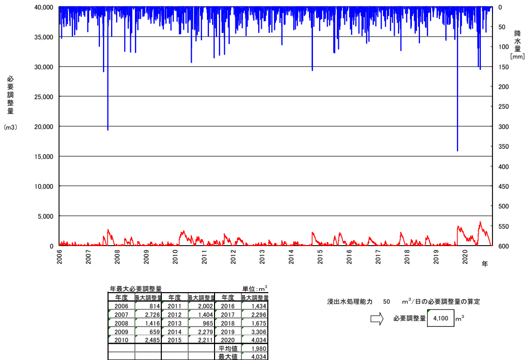
図 3-65 処理能力及び調整槽容量の算定結果（案 2）
