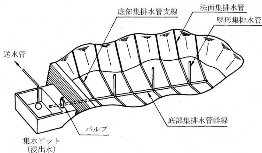
図 3-71 浸出水集排水設備の概念図
