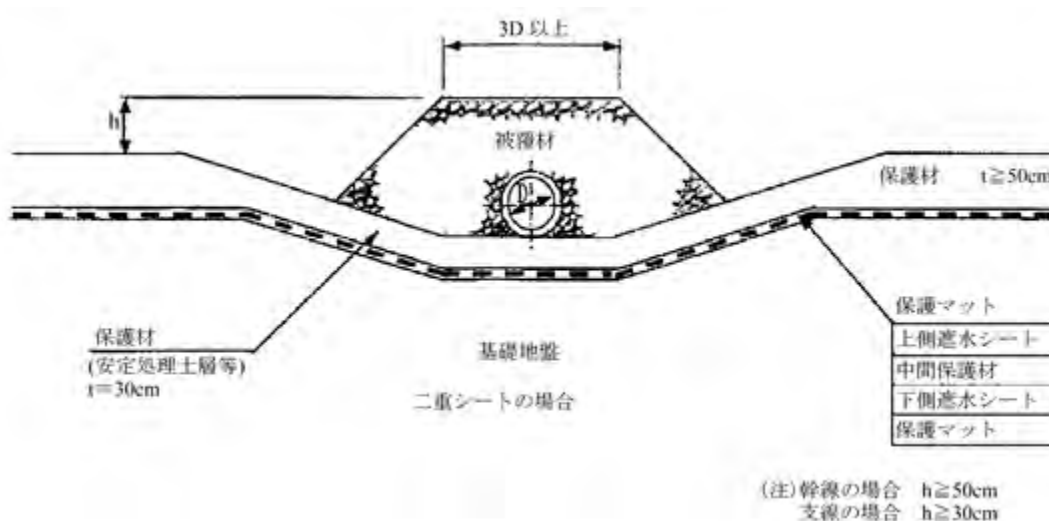
図 3-72 底部集排水管の構造例
