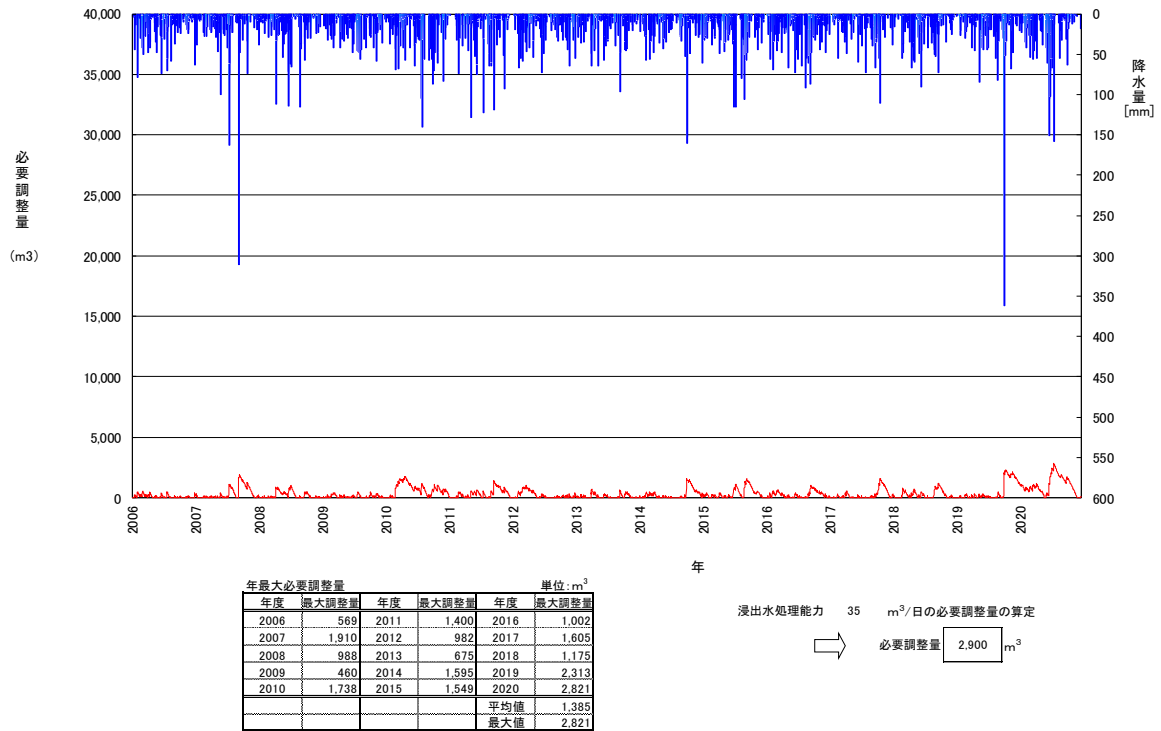
図 3-66 処理能力及び調整槽容量の算定結果（案 3）
