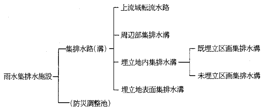
図 3-70 雨水集排水施設の概念図
