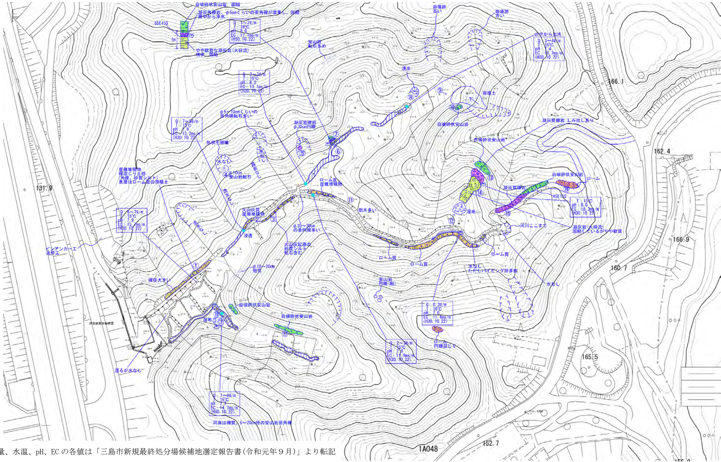
図 3-46 地質踏査図
