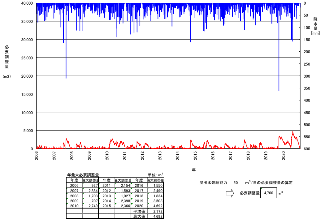
図 3-64 処理能力及び調整槽容量の算定結果（案 1）
