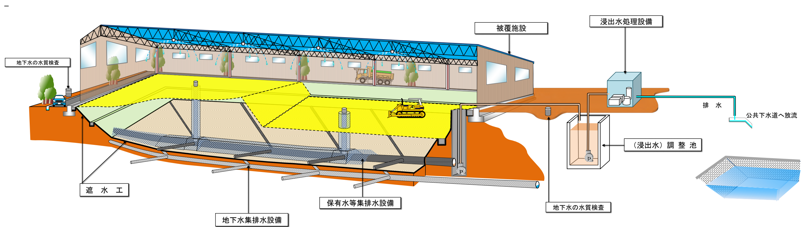
図 3-1 オープン型埋立地と被覆型埋立地のイメージ図
