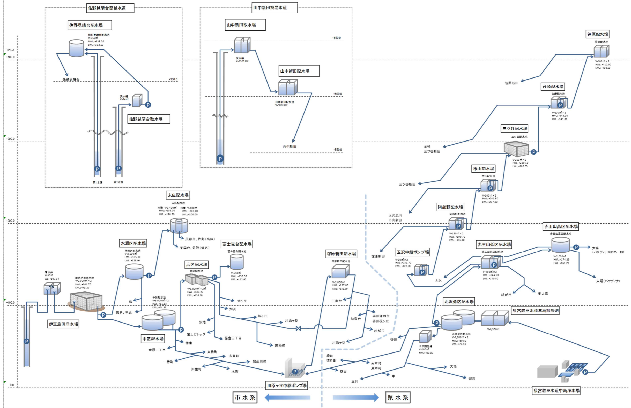
図1 三島市水道施設フロー図
